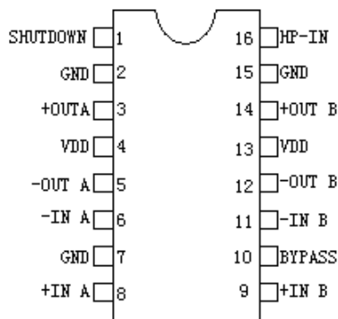
SOP16 (DIP16)
