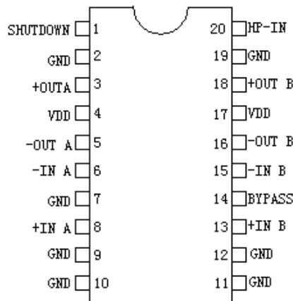
TSSOP20
